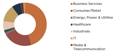
Branschfördelning
