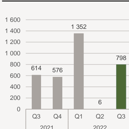
Projektförvärv, MW
