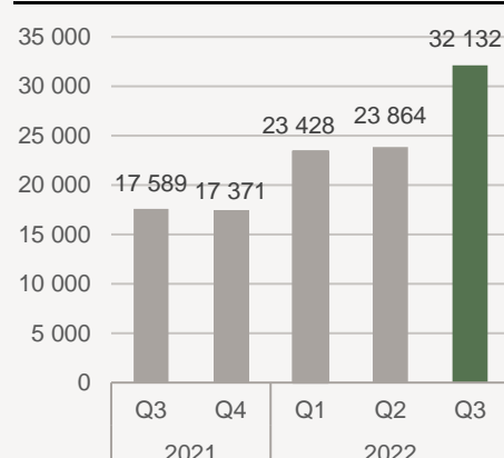
Projektutvecklingsportfölj, MW
