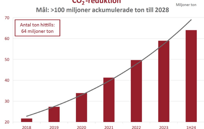
CO 2 -reduktion
