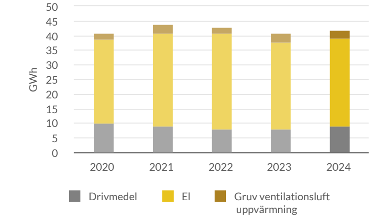
Bild 5. Energiförbrukning, Gigawattimmar (GWh).
