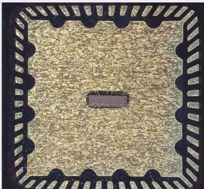
Et mislykket forsøk på å trådlodde I/O for AI-delen.
