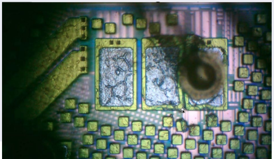
Fotografi som viser hvor lite feilmargin vi har for trådlodding av enkelte I/O-pads.
