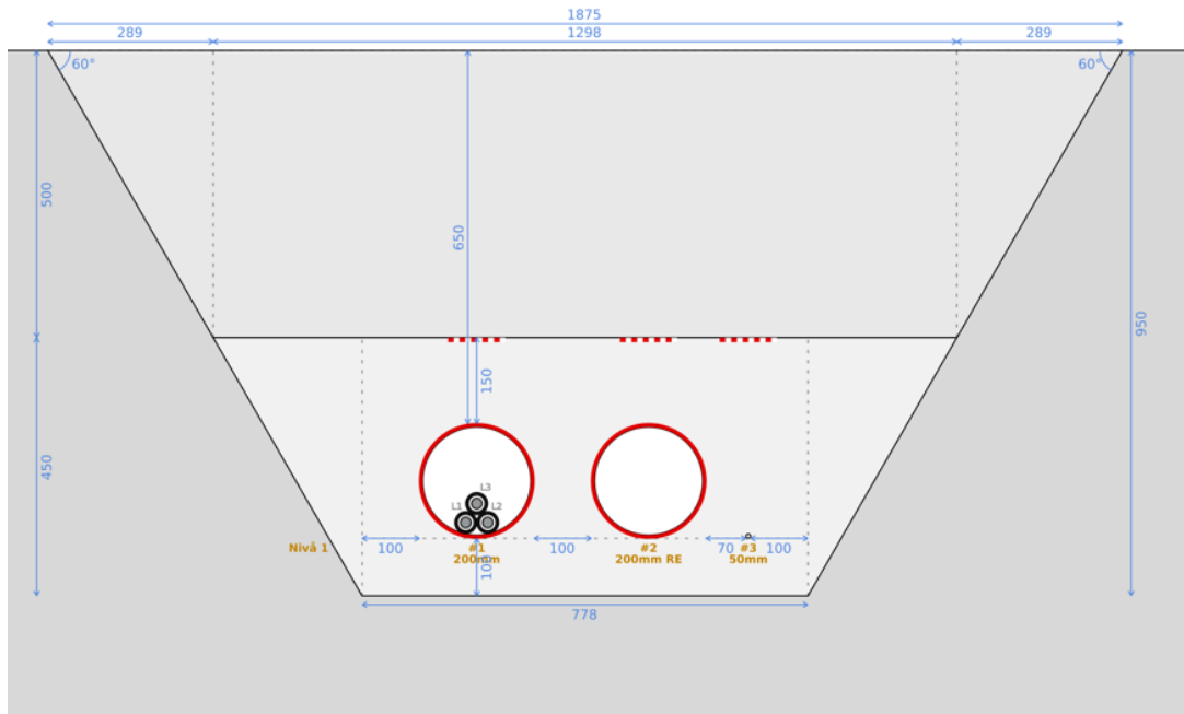
Figur 3-8. Typisk grøftesnitt for 11 kV kabler.
