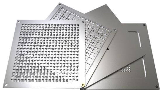
Gapwaves gapvågledarantenn
