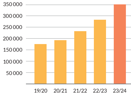
Nettoomsättning, tkr
