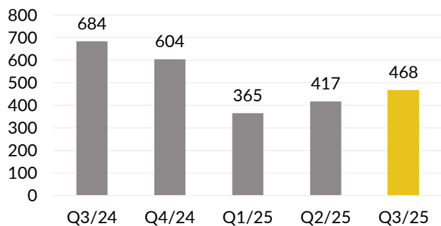
Guldproduktion, oz
