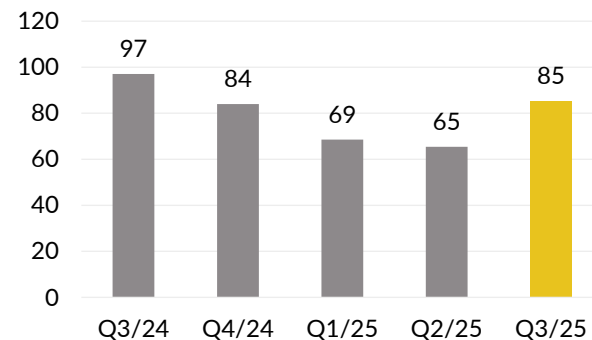
Zinkproduktion, ton
