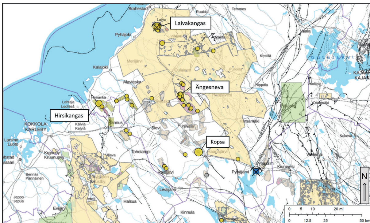
FIGURE 2: KARTA ÖVER MELLANÖSTERBOTTNISKA GULDBÄLTET.
