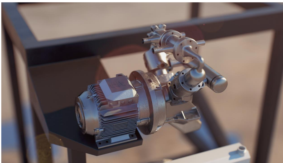
Azelios Stirlingmotor. Motorn drivs av värme från det termiska energilagret för produktion av förnybar el under dygnets alla timmar, med hög effektivitet och helt utan utsläpp.
